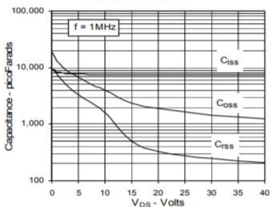
Fig. 11. Capacitance
