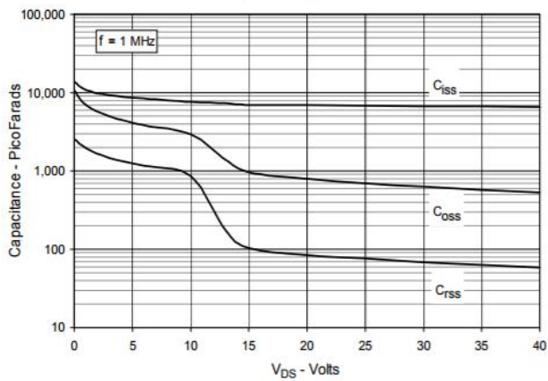
Fig. 11. Capacitance
