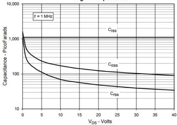
Fig. 11. Capacitance
