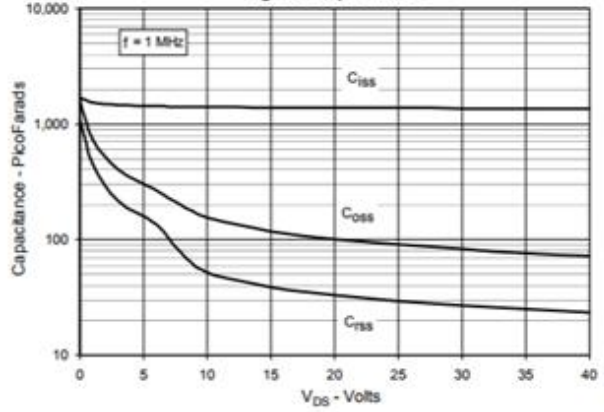
Fig. 10. Capacitance
