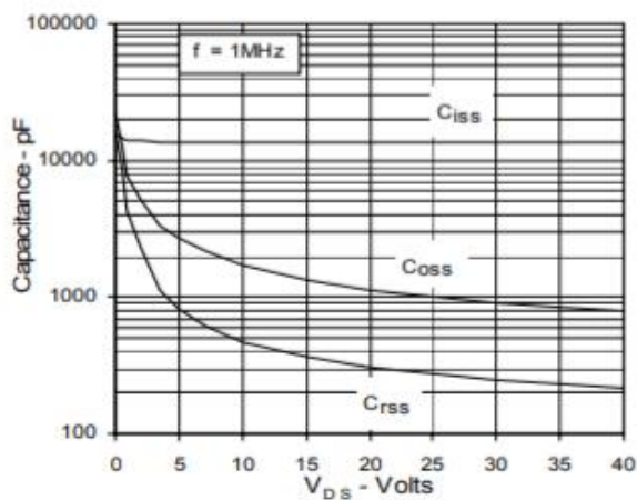
Fig. 11. Capacitance
